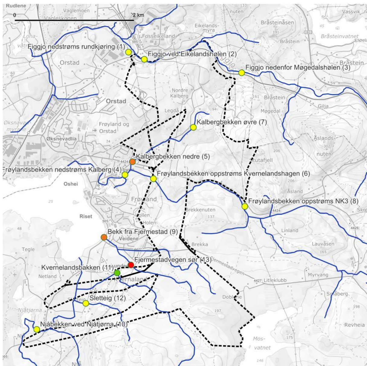
Figur 5.1. Samlet økologisk tilstand ved overvåkingsstasjoner basert på overvåkingsdata av bunndyr og vannkjemi innsamlet høst 2023 og vinter/vår 2024. Grønn = god tilstand, gul = moderat tilstand, oransje = dårlig tilstand, rød = svært dårlig tilstand.
