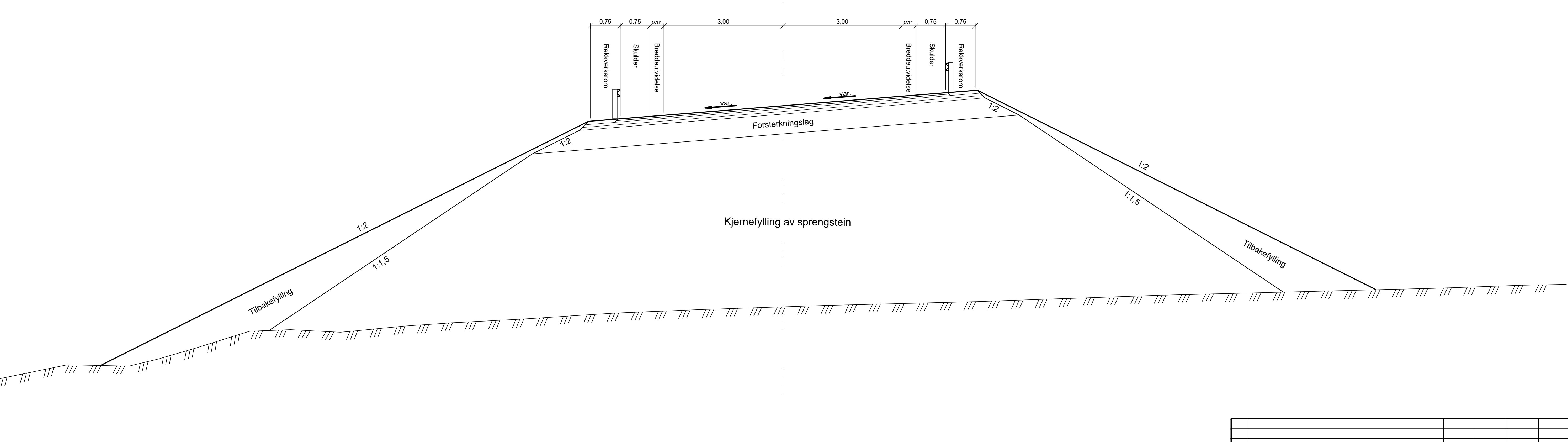
Veg. Undergrunn T2; steinfylling vmød 11.000
