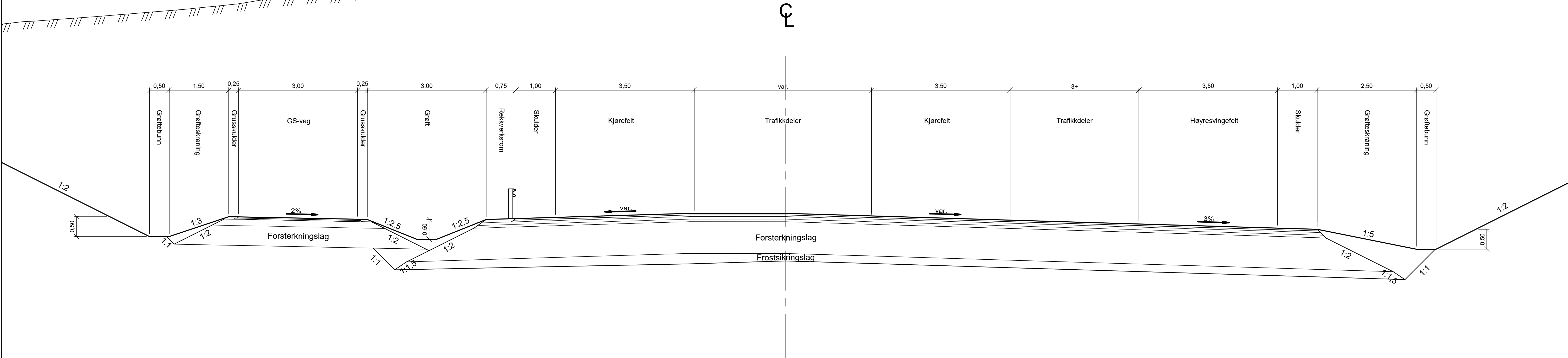
Veg m. høyresvingefelt og gs-veg. Undergrunn T4; jordskjæring vmød 10.000
