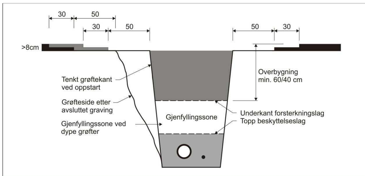
Normalprofil av grøft i vei
