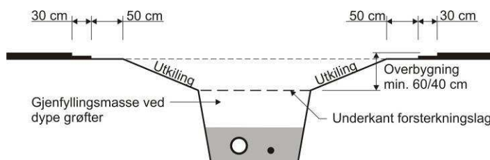
Utrasing av grøfteside. Her må det foretas skjæring av asfalt og justering av grøfteskråning
