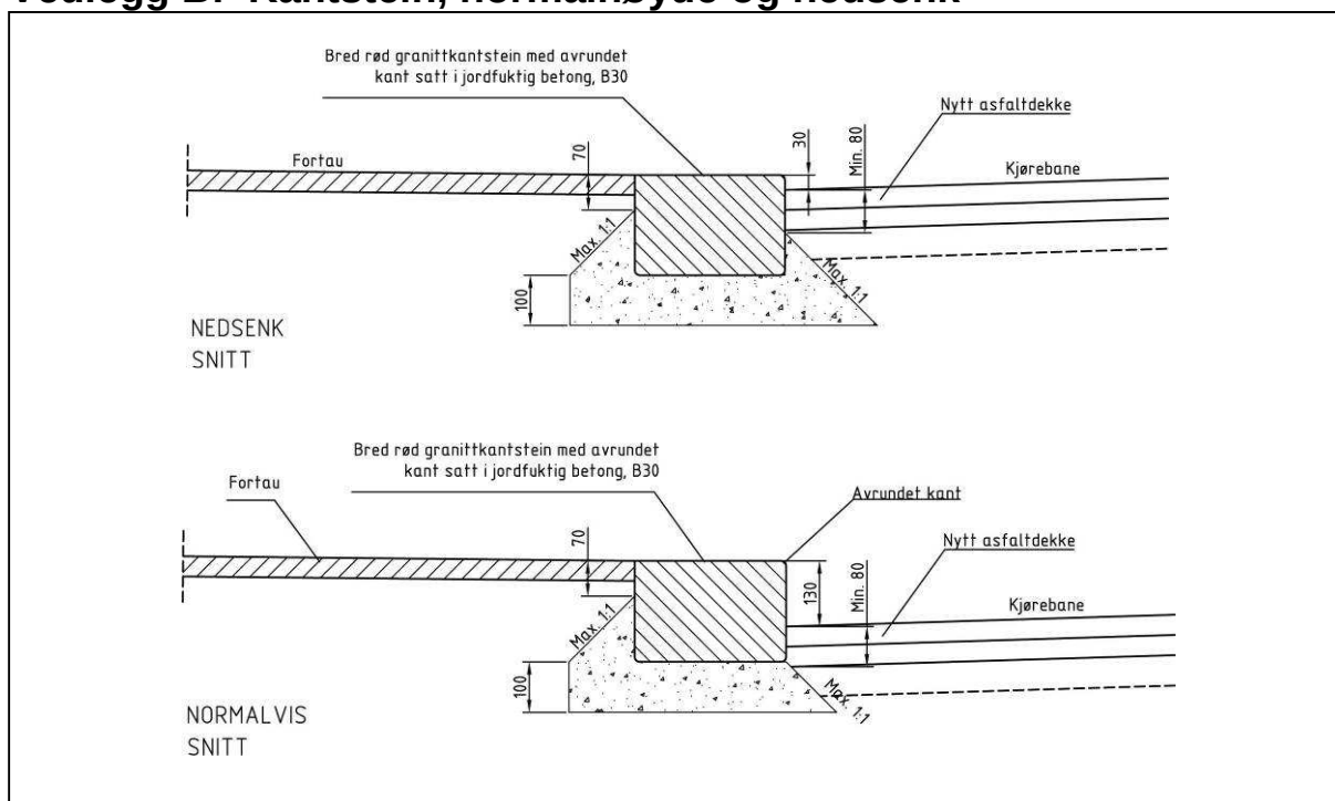
Detalj bred kantstein uten renne
