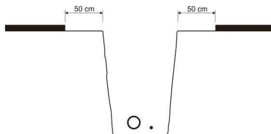
Skjæring for planlagt grøft i asfaltert areal.
