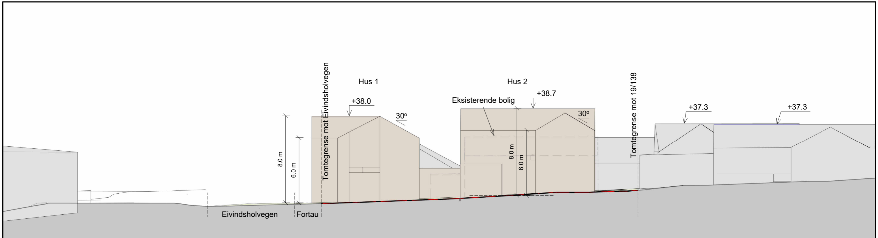
T1 1 : 200
